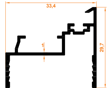
Sabit Cam Kilit Karşılığı Profil Stable Glass Lock Prevention Profile
