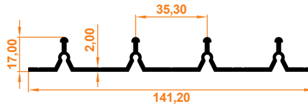
Dörtlü Eşiksiz Alt Kasa Profil Quadruple Lower Case Profile Thresholdless
