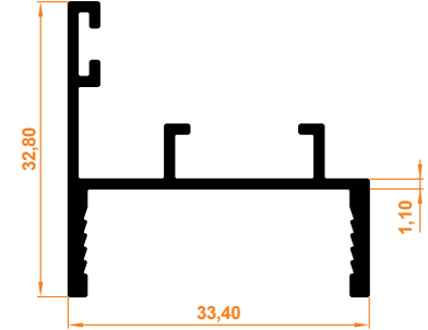
Sabit Cam İspanyolet Karşılık Profil Fixed Glass Espagnolette Handle Provision Profile
