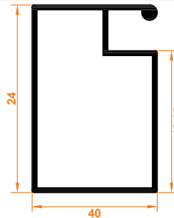
17x25 Sineklik 17x25 Fly Screen
