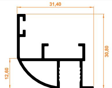
8 mm İspanyollet Profil Karşılığı 8 mm Espagnolette Combination Profile
