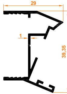
22,5° Dönüş Profil 22,5° Return Profile
