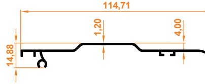
Küpeşte Profil Handrail Profile
