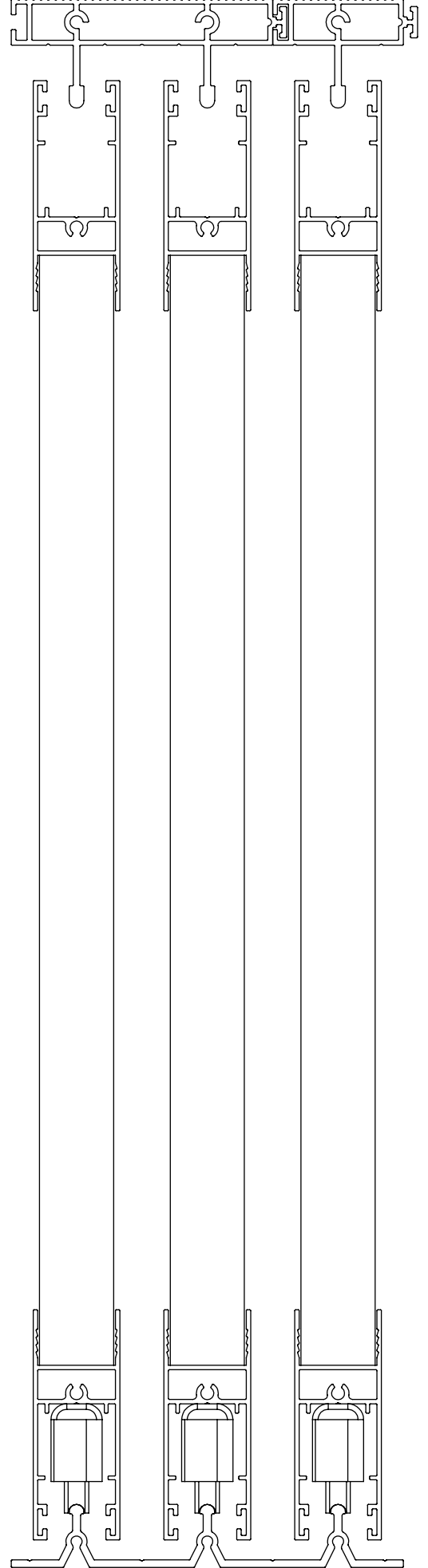
Eşiksiz Sistem Thresholdless System
