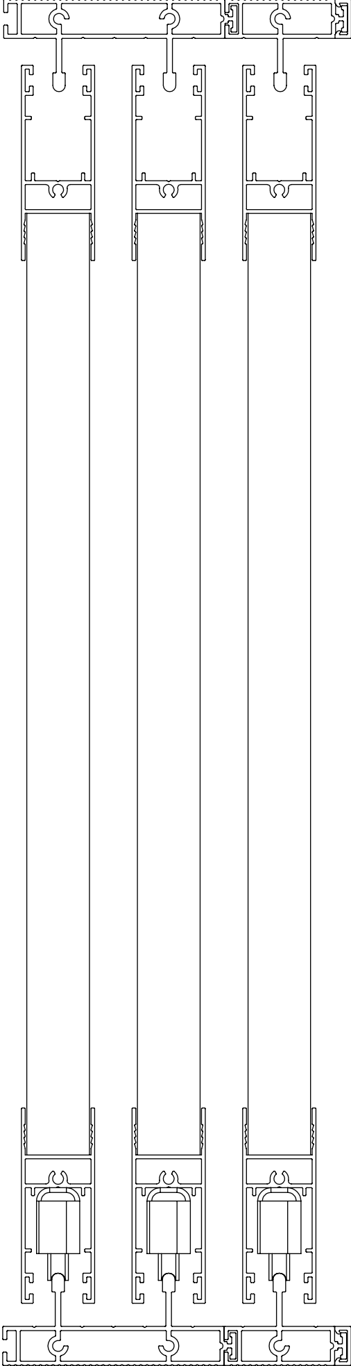
Eşikli Sistem Threshold System
