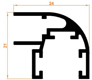
Köşe Dönüş Fitil Corner Return Wick
