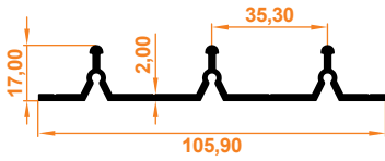
Üçlü Eşiksiz Alt Kasa Profil Triple Lower Case Profile Thresholdless
