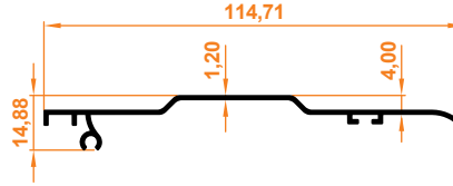
Küpeste Profil Handrail Profile
