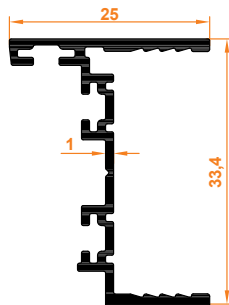
Sabit Cam Menteşe Profil Stable Glass Hinge Profile
