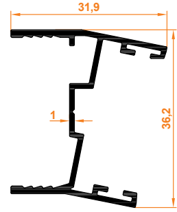
11° Dönüş Profil 11° Return Profile
