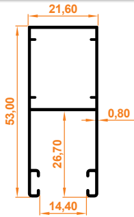
39'lik Yan Dikme 39 Side Column
