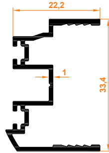
Açılı Dönüş Menteşe Profil PopUp Return Hinge Profile
