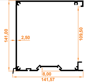
Üst Kasa Profil Top Case Profile
